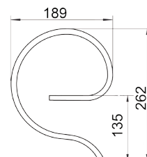
WZMOCNIENIE ZĘBA SPRĘŻYNOWEGO • STRENGTHENING OF S-TINE • VERSTÄRKUNGS FEDER 32x12 1417/00-001/1
