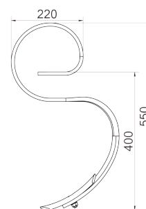
ZĄB SPRĘŻYNOWY Z REDLICZKĄ · SPRING S-TINE WITH CULTIVATOR POINT · FEDERZINKEN MIT SCHAR 32x10 1417/00-003/0
