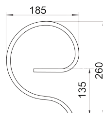
WZMOCNIENIE ZĘBA SPRĘŻYNOWEGO • STRENGTHENING OF S-TINE • VERSTÄRKUNGS FEDER 32x10 1417/00-001/0
