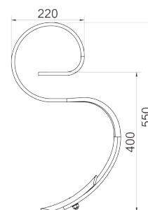
ZĄB SPRĘŻYNOWY Z REDLICZKĄ · SPRING S-TINE WITH CULTIVATOR POINT · FEDERZINKEN MIT SCHAR 32x12 1417/00-002/0
