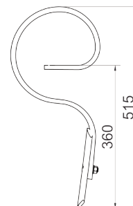
ZĄB PROSTY DUŃSKI Z REDLICZKĄ • DUNISH STRAIGHT TINE WITH CULTIVATOR POINT • DÄNISCHER GAREZINKEN, GERADE 32x10 1417/00-003/2
