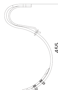
ZĄB KULTYWATORA Z REDLICZKĄ CULTIVATION TINE WITH CULTIVATOR POINT KULTIVATOR-ZINKEN MIT SCHAR 40x10 1410/01-001/0
