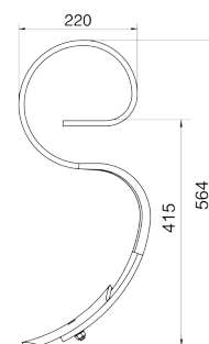
ZĄB TYPU SU Z REDLICZKĄ · TINE-SU WITH CULTIVATION POINT · FEDERZINKEN DES SU-TYPS 32x10 1680/00-500/1
