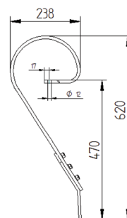
ZĄB SPRĘŻYNOWY Z PŁASKĄ REDLICĄ • TINE WITH FLAT CULTIVATION POINT • FEDERZINKEN 45x10 3074/00-041/0
