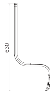
ZĄB SIEWNIKA „Z” Z REDLICZKĄ · TINE SEEDER TYPE „Z” · SPURLOCKERER „Z” MIT SCHAR 32x10 3074/00-042/0
