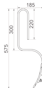
ZĄB SPRĘŻYNOWY SIEWNIKA Z REDLICZKĄ · SPRING TINE SEEDER WITH CULTIVATOR POINT · SPURLOCKERER MIT SCHAR 32x10 3074/00-041/0
