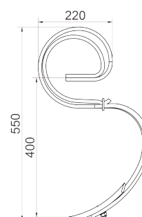
ZĄB SPRĘŻYNOWY WZMOCNIONY Z REDLICZKĄ · SPRING S-TINE WITH CULTIVATOR POINT · VERSTÄRKTER FEDERZINKEN 32x12 1417/00-005/0
