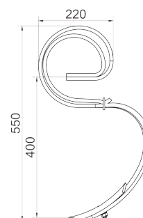
ZĄB SPRĘŻYNOWY WZMOCNIONY Z REDLICZKĄ · SPRING S-TINE WITH CULTIVATOR POINT · VERSTÄRKTER FEDERZINKEN 32x10 1417/00-004/0
