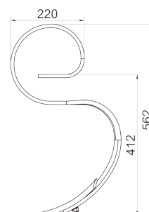
ZĄB SPRĘŻYNOWY Z REDLICZKĄ • SPRING S-TINE WITH CULTIVATOR POINT • FEDERZINKEN MIT SCHAR 32x10 1767/10-400/1
