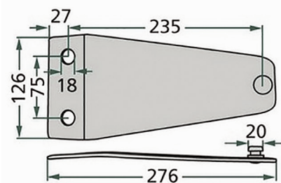
TRZYMAK NOŻA • MOWER BLADE HOLDER • MESSERHALTER 3.525PZ-0116 DEUTZ FAHR • KVERNELAND • PZ • VICON • TAARUP • ZWEEGERS
